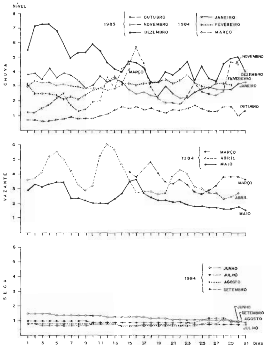
Fig. 2. Flutuações sazonais do nível do rio Cuiabá, em Cuiabá. Fonte: Agência da Capitania dos Portos em Cuiabá - MT.
