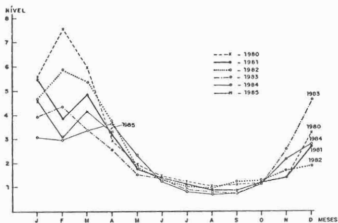
Fig. 1. Distribuição mensal das médias de altura do nível do rio Cuiabá, em Cuiabá. Fonte: Agência da Capitania dos Portos em Cuiabá - MT.
